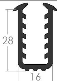
B48 – Uszczelka dwustronna szybowa (8,6/16/28)
