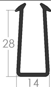
B49 – Uszczelka dwustronna szybowa (10,6/14/28)
