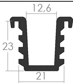
B61 – Uszczelka dwustronna szybowa (12,6/21/23)
