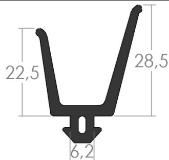
N305 – Uszczelka wargowa 6,2
