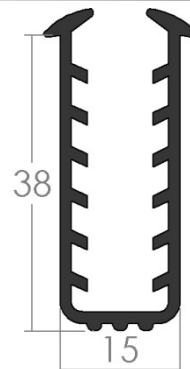
B59 – Uszczelka dwustronna szybowa (8,3/15/38)
