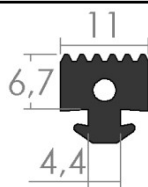
N301 – Uszczelka podszybowa 4,4/6,7 (10/*/*)
