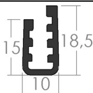
N252 – Uszczelka podszybowa (5,2/10/15-18,5)
