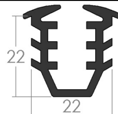
B56 – Uszczelka dwustronna szybowa (8,1/22/23)
