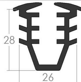
B57 – Uszczelka dwustronna szybowa (8,1/26/28)
