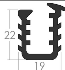
B55 – Uszczelka dwustronna szybowa (8,6/19/22)
