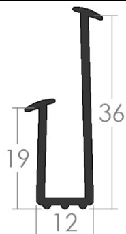
B60 – Uszczelka dwustronna szybowa (8,6/12/19-36)
