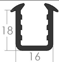
B47 – Uszczelka dwustronna szybowa (10,6/16/18)
