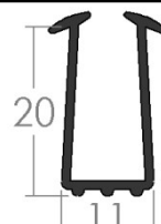
B58 – Uszczelka dwustronna szybowa (8,6/11/20)
