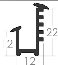
B41-2 – Uszczelka szybowa (6/12/22-12)
