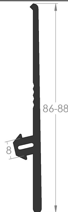
N306-2 – Uszczelka okapnikowa
